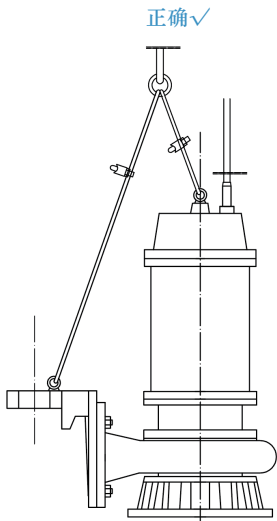
通过短链条将泵调整至竖直状态
