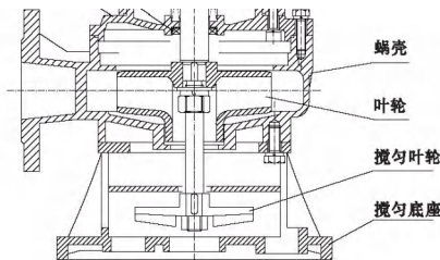
搅匀底座结构图
