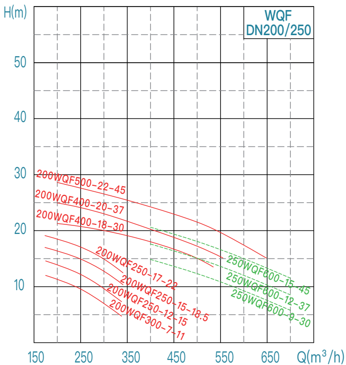
WQF系列性能曲线图 50Hz
