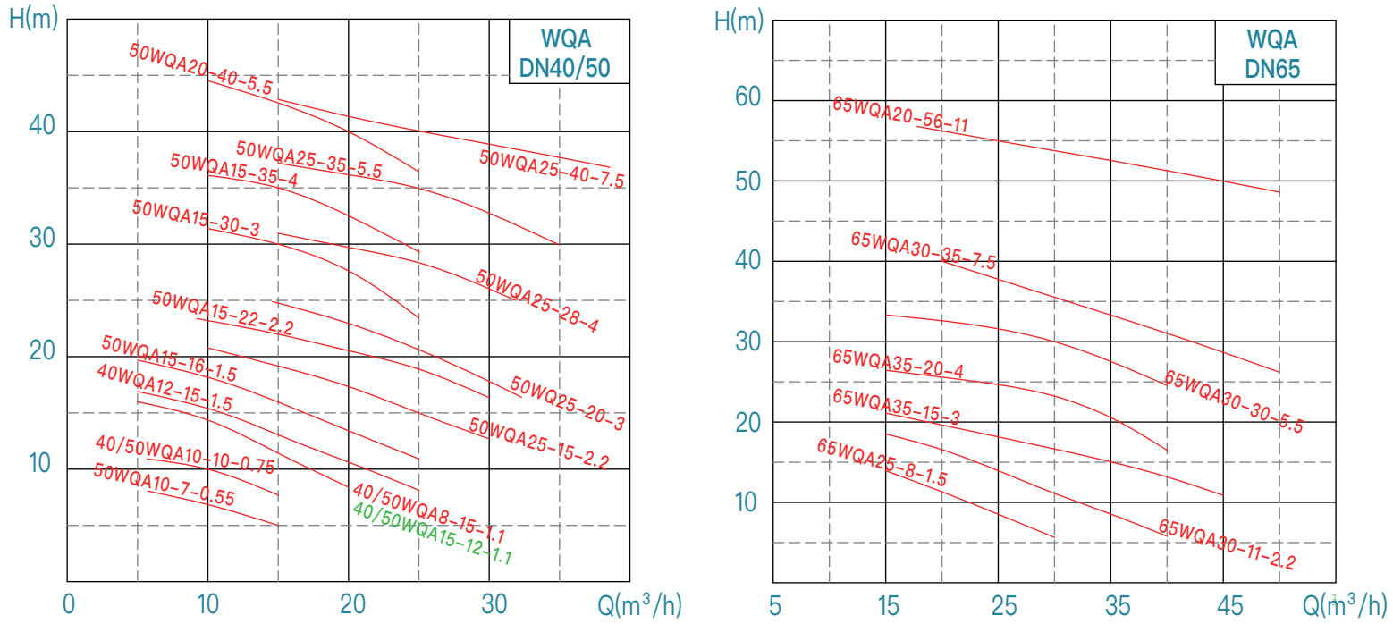
WQA系列性能曲线图 50Hz
