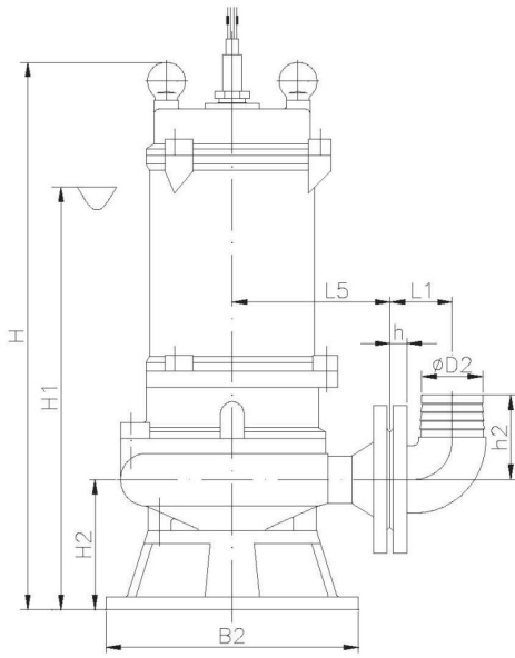
软管（弯头）移动式安装
