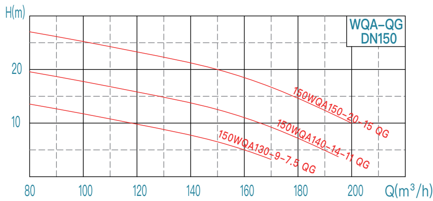
WQA-QG系列 性能曲线图 50Hz
