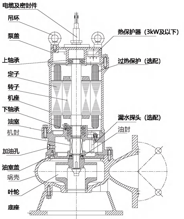
7.5 kW 及以下结构图
