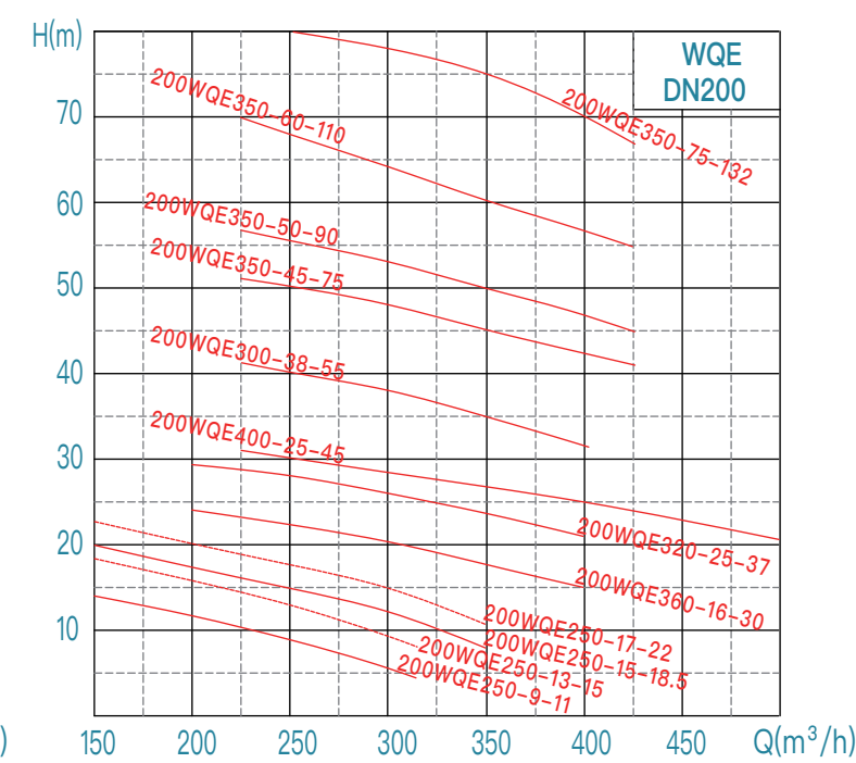
WQE系列性能曲线图 50Hz
