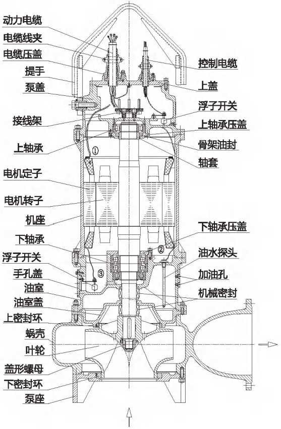
11 kW-4P 及以上结构图
