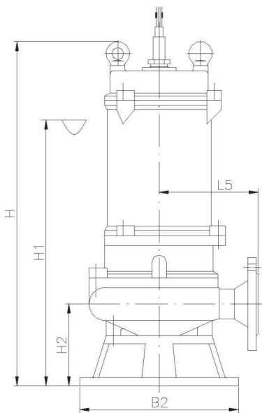
泵外形尺寸图
