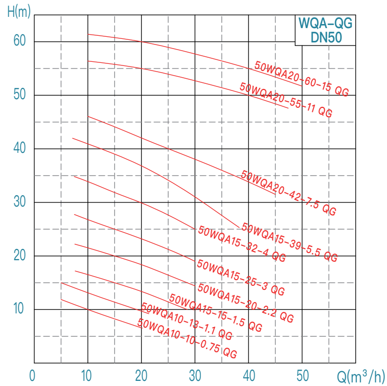
WQA-QG系列 性能曲线图 50Hz
