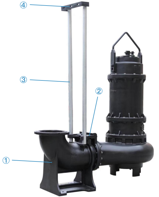
自动耦合安装结构图
