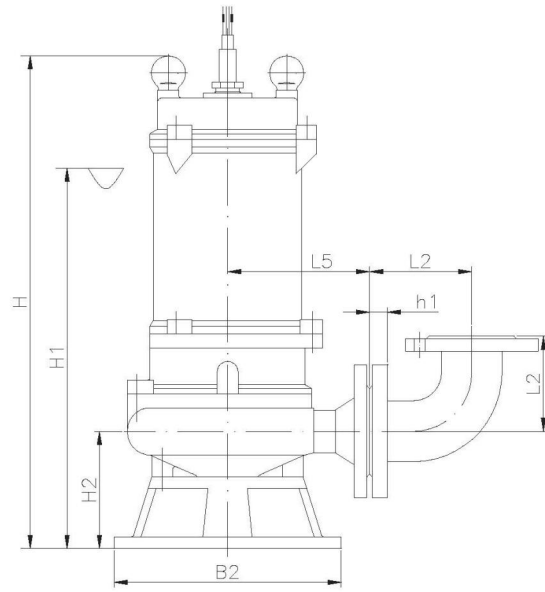
硬管（双法兰弯头、弯接）移动式安装
