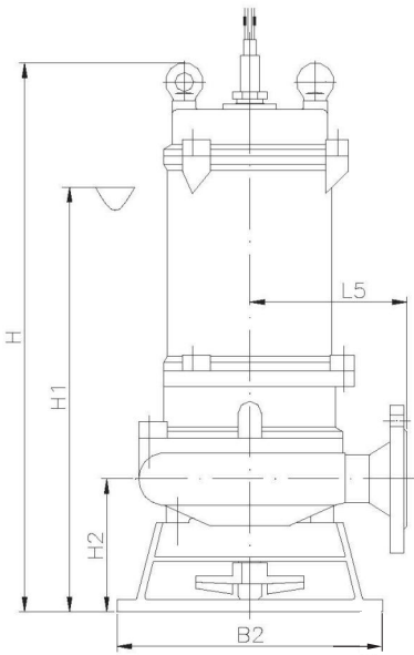
搅匀 (JY) 泵外形尺寸图
