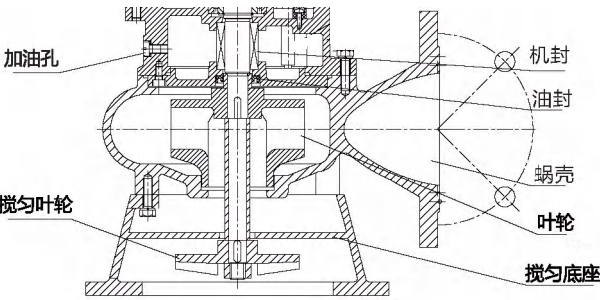
搅匀底座 结构图
