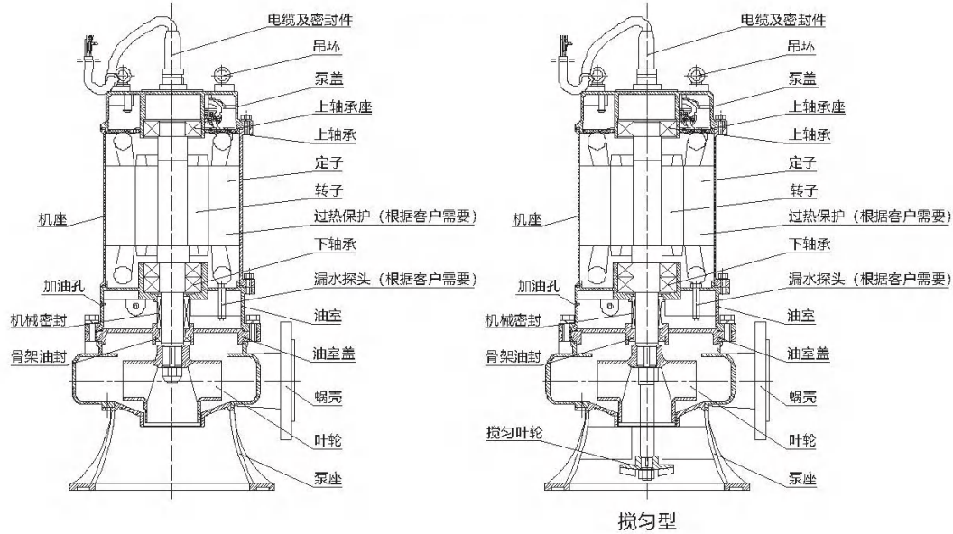
7.5 kW 及以下结构图
